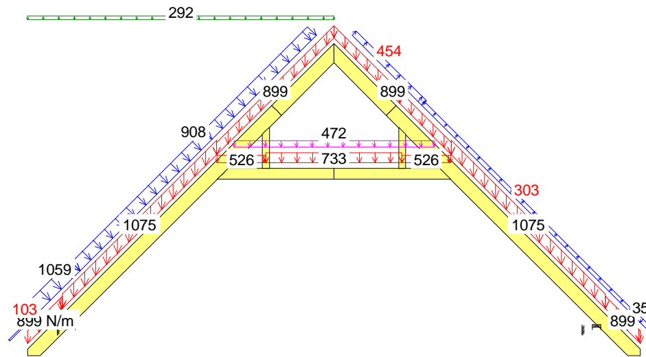
16 Kr 1.15*Stałe+1.05*(OZ1+OZ2+OZ3)+0.75*ŚniegL(OP)+1.5*WiatrL
