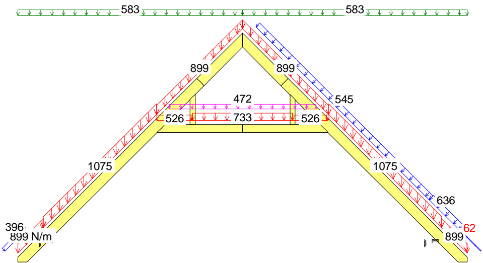
10 Kr 1.15Stale+1.5Śnieg+1.05(OZ1+OZ2+OZ3)+.9WiatrP(brakssania)
