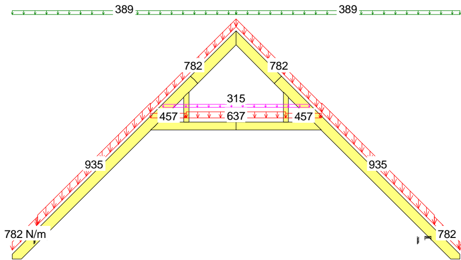
18 Śr Stałe + Śnieg + 0.7*(OZ1 + OZ2 + OZ3), Winst
