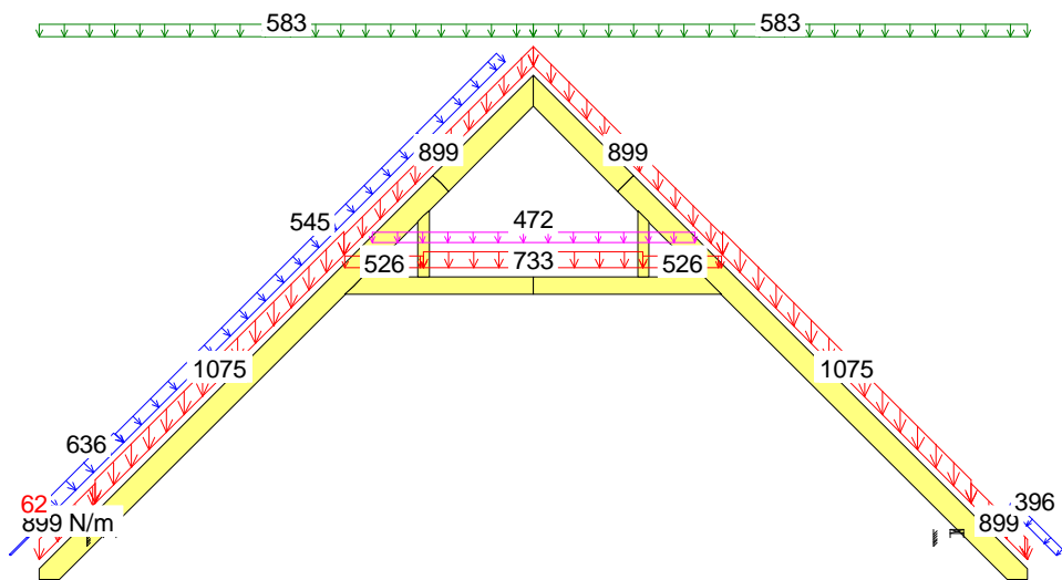
9 Kr 1.15Stale+1.5Śnieg+1.05(OZ1+OZ2+OZ3)+.9WiatrL(brakssania)
