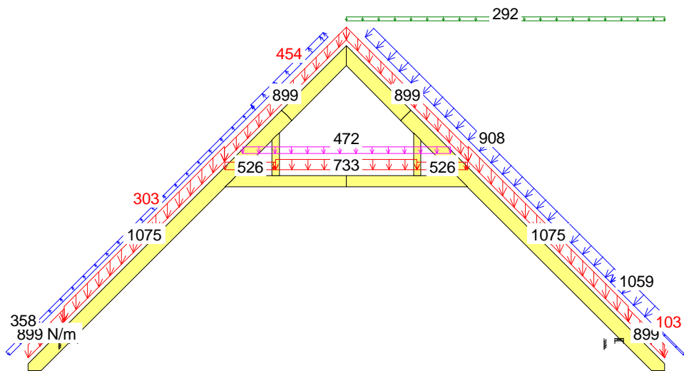
17 Kr 1.15*Stałe+1.05*(OZ1+OZ2+OZ3)+0.75*ŚniegP(0L)+1.5*WiatrP
