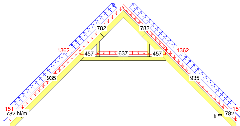
11 Kr Stale + 1.5*Wiatr na szczyt
