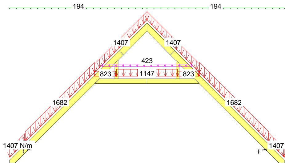
25 Śr 1.8 \cdot \text{Stale} + 0.5 \cdot \text{Śnieg} + 1.24 \cdot \text{OZ2 inne poł.} + 0.94 \cdot (\text{OZ1} + \text{OZ3}) , Wfin
