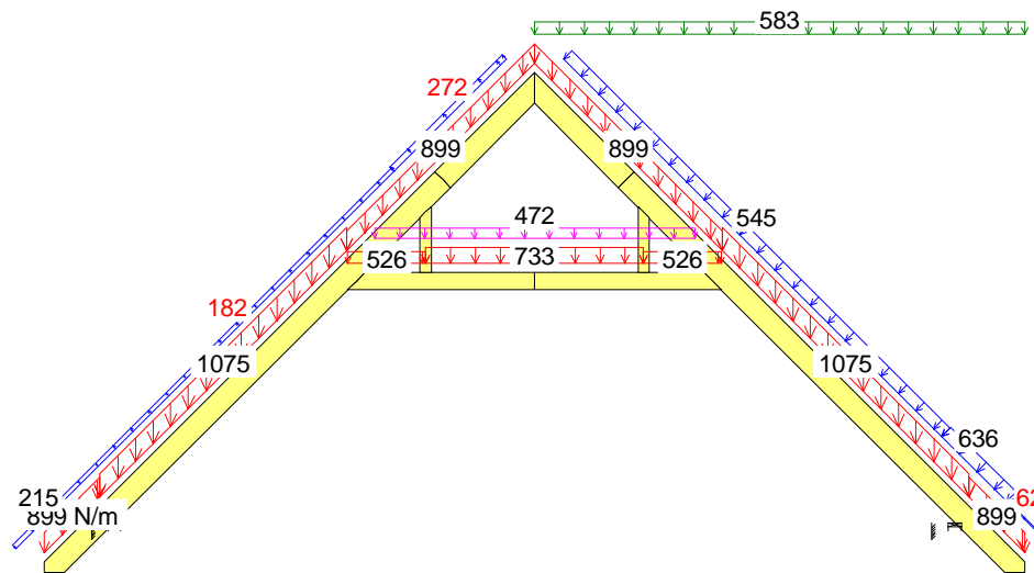
15 Kr 1.15*Stałe+1.05*(OZ1+OZ2+OZ3)+1.5*ŚniegP(OL)+0.9*WiatrP
