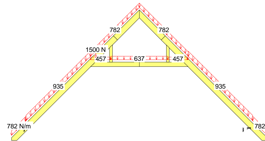
12 Ch Stale + 1.5*Człowiek na lewym PG
