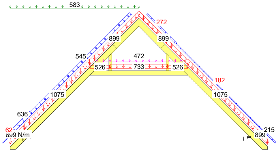
14 Kr 1.15*Stałe+1.05*(OZ1+OZ2+OZ3)+1.5*ŚniegL(OP)+0.9*WiatrL
