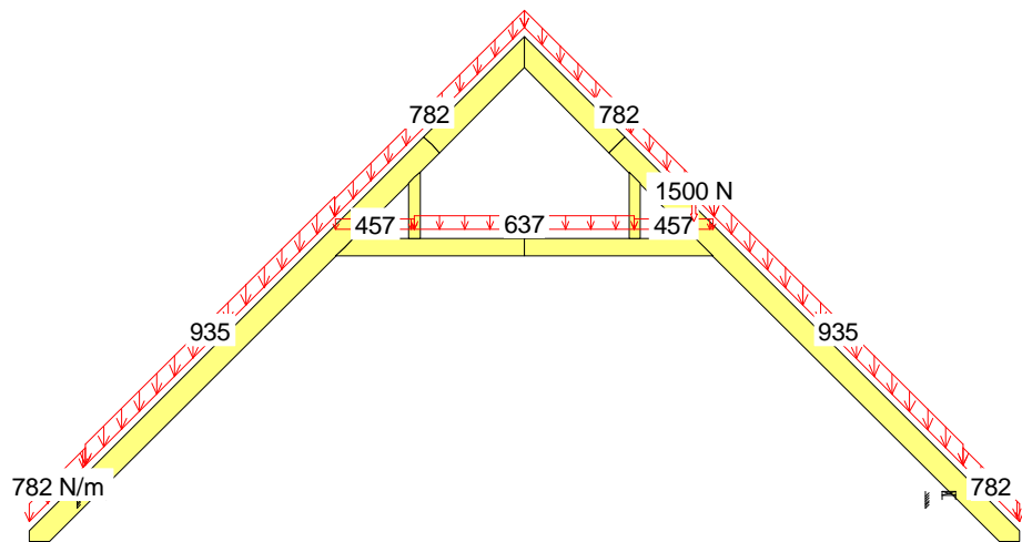
13 Ch Stałe + 1.5*Człowiek na prawym PG
