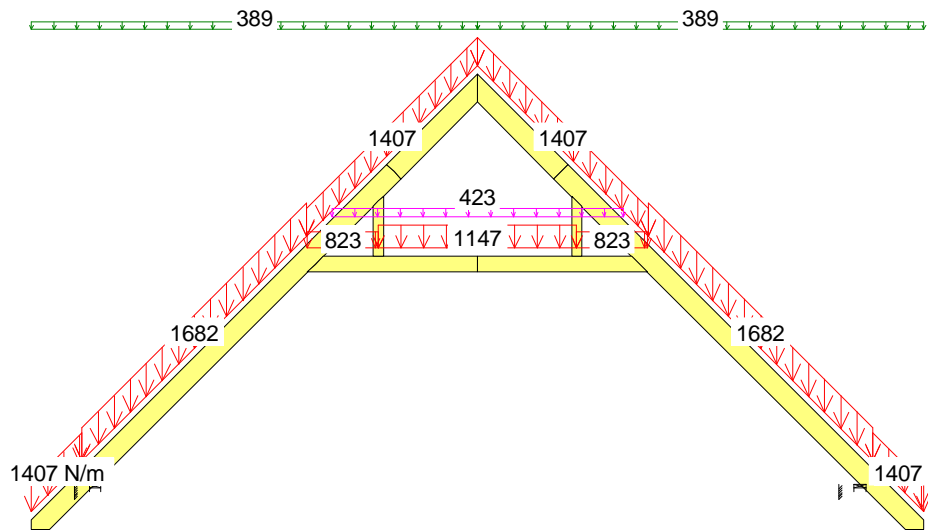
19 Śr 1.8*Stałe + Śnieg + 0.94*(OZ1 + OZ2 + OZ3), Wfin
