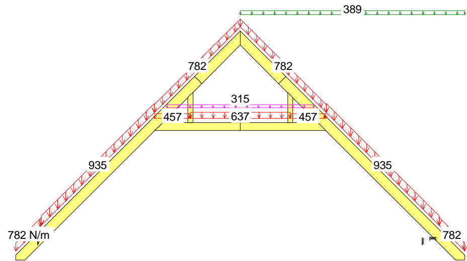
20 Śr Stałe + ŚniegP(0L) + 0.7*(OZ1 + OZ2 + OZ3), Winst
